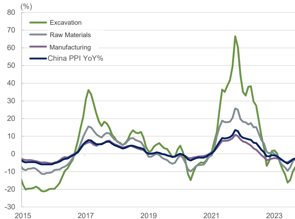
PPIの推移
