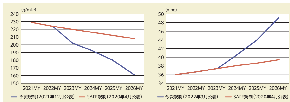
図表1. GHG規制(左側)、CAFE規制(右側)の基準値
